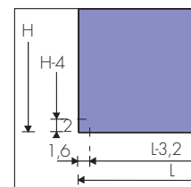
SO-FLEX-FXV 77 - ... ▲▽ t. c.= L-3,2 cm
