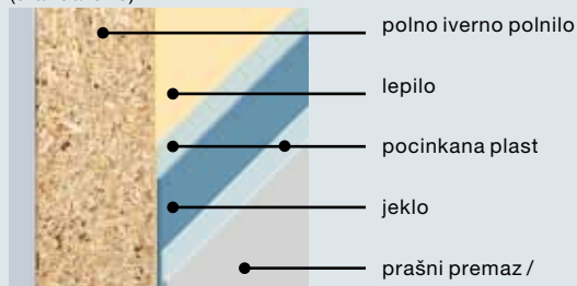
Polno iverno polnilo (po naročilu) za boljšo protihrupno zaščito
