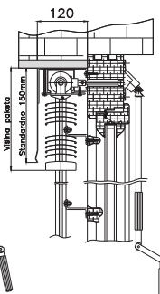
Montaža z 90° zglobom
