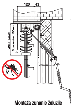
Montaža zunanje žaluzije s komarnikom
