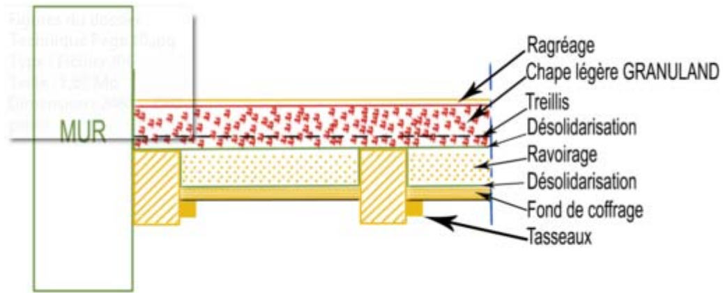
Figure 1 – Coffrage porteur entre solives
