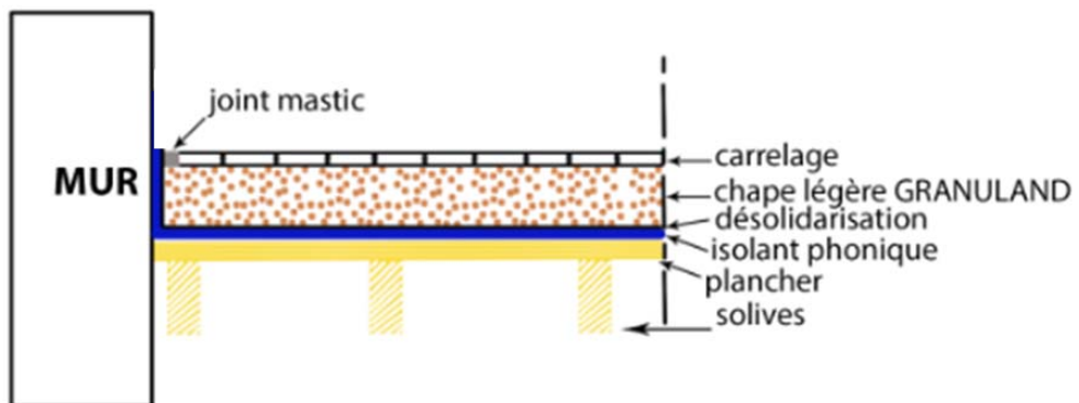
Figure 6 – Joint mastic en périphérie pour local E2
