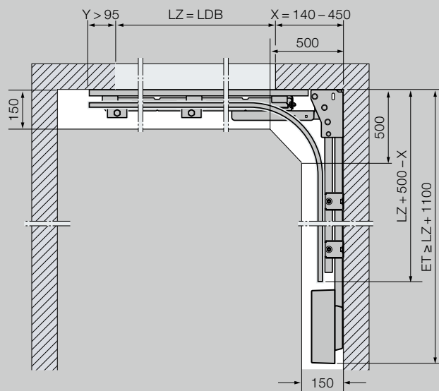
Okovje DS (dvojno vodilo) pogon za stensko montažo
