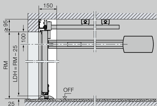
Okovje ES (enojno vodilo) pogon za stensko montažo
