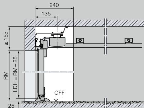
Okovje ES (enojno vodilo) pogon za stropno montažo A
