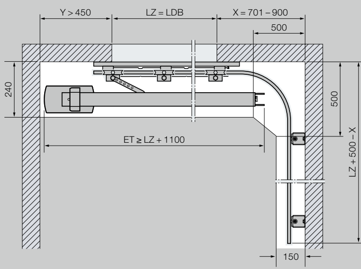
Okovje ES (enojno vodilo) pogon za stropno montažo B
