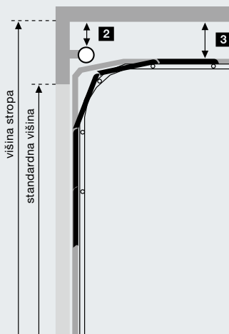
2 Potreben prostor za sekcijška garažna vrata s tehniko torzijskih vzmeti
