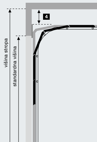
4 Potreben prostor za sekcijška garažna vrata s tehniko torzijskih vzmeti
