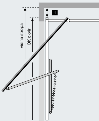
1 Potreben prostor za Berry dvižna vrata
