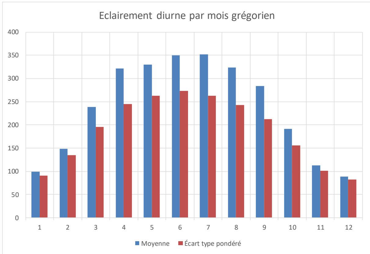
Figure 10 : Éclairage solaire diurne : moyenne et écart-type par mois grégorien
