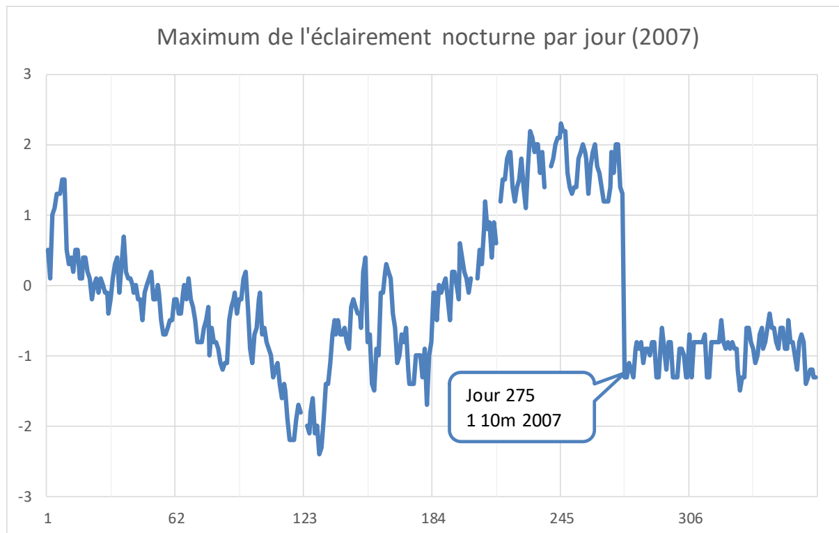
Figure 5 : Maximum d'éclairement nocturne par jour en 2007
