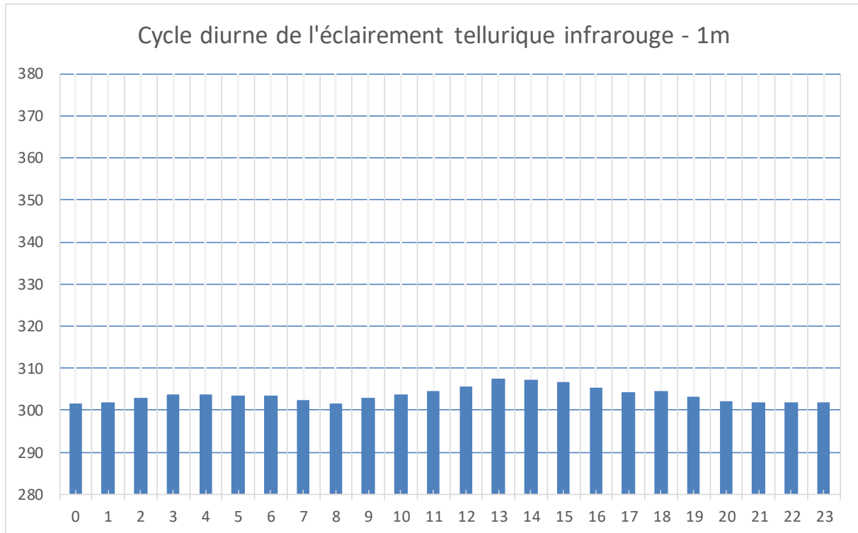
Figure 32 : Cycle diurne de l'éclairage tellurique en unème
