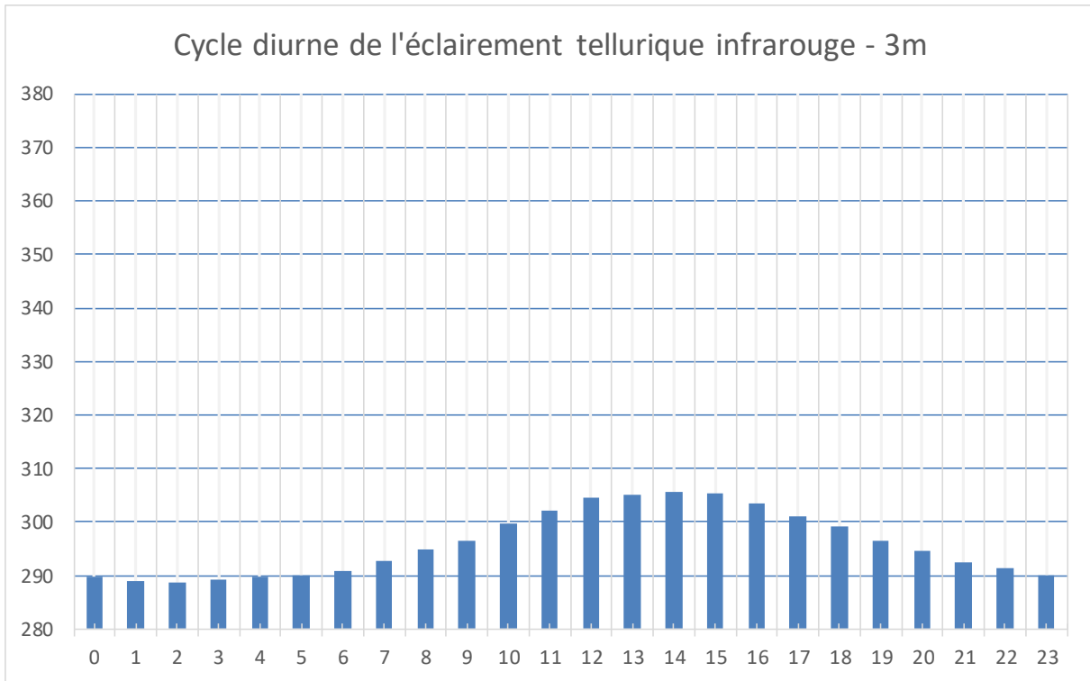
Figure 34 : Cycle diurne de l'éclairage tellurique en tertème
