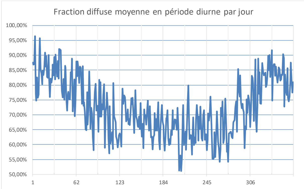
Figure 23 : Fraction diffuse moyenne de l'éclairement en période diurne, par jour
