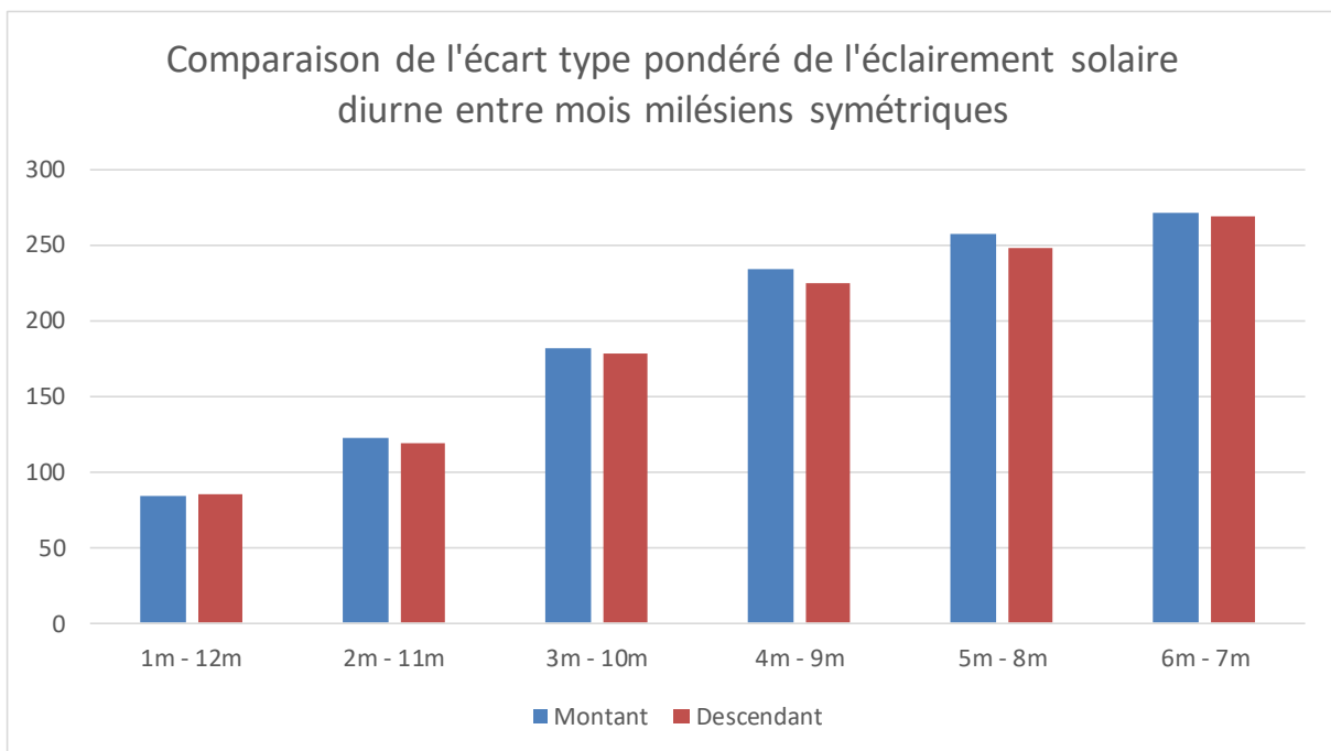
Figure 13 : Comparaison de l'écart-type pondéré de l'éclairement entre mois milésiens
