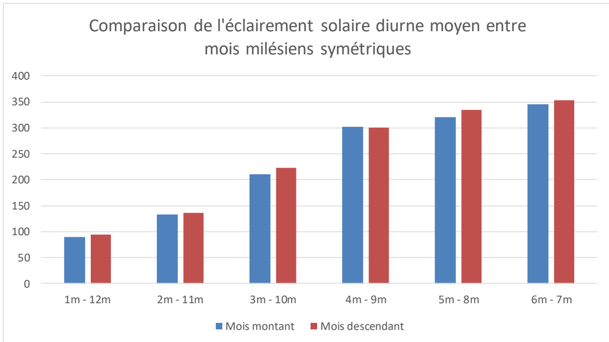
Figure 12 : Comparaison de l'éclairement solaire diurne moyen entre mois symétriques
