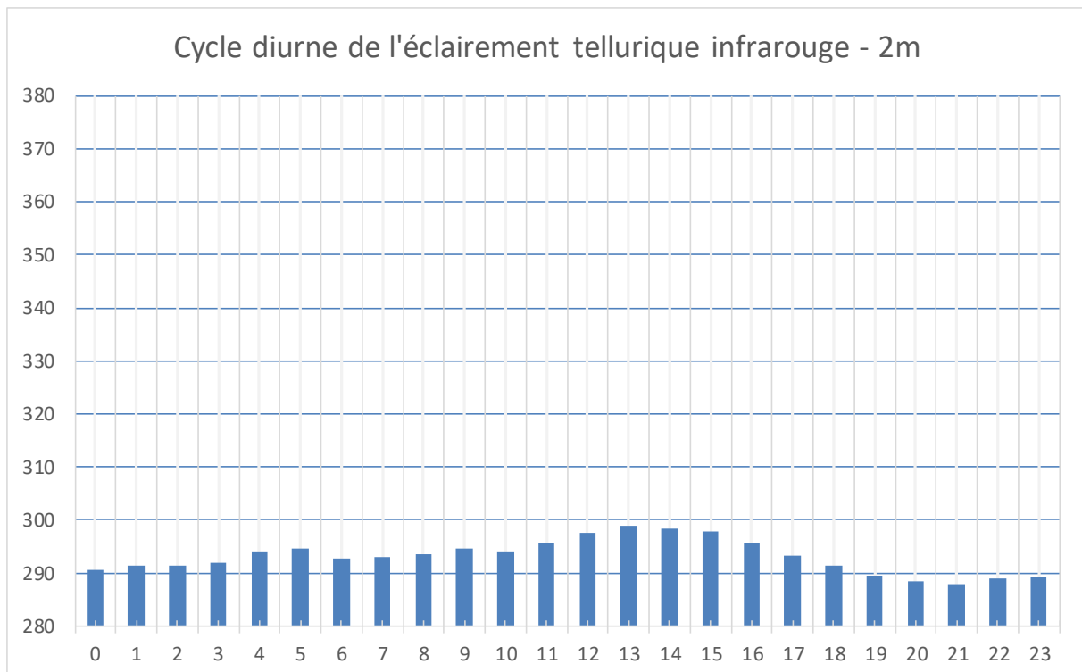
Figure 33 : Cycle diurne de l'éclairage tellurique en secondème
