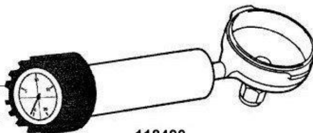
118490 Prüfsiebträger zur Druckprüfung an der Gruppe
